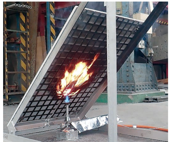
延焼性試験状況 (HM-C22) NEXCOはく落対策工の延焼性・自己消火性規定値を満足しています
