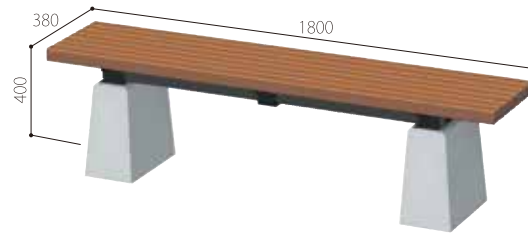
品番:DLB-50*45-FLAT-PC サイズ: W380×L1800×H400 標準価格 164,000円/基(税抜)
