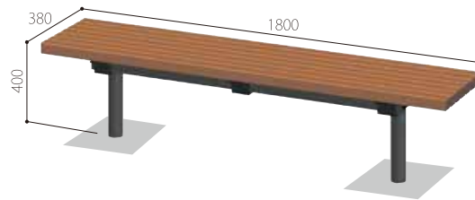
品番:DLB-50*45-FLAT サイズ: W380×L1800×H400 標準価格 119,000円/基(税抜)
