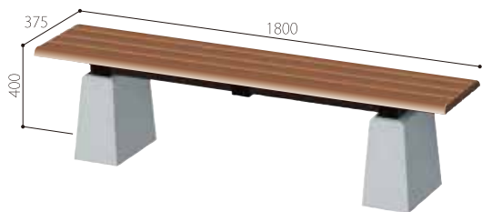
品番:DLB-90*40R-FLAT-PC サイズ: W375×L1800×H400 標準価格 105,000円/基(税抜)
