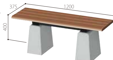
品番:DLB-90*40R-FLAT*1200-PC サイズ: W375×L1200×H400 標準価格 93,000円/基(税抜)
