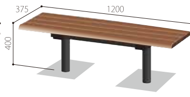
品番:DLB-90*40R-FLAT*1200 サイズ: W375×L1200×H400 標準価格 81,000円/基(税抜)
