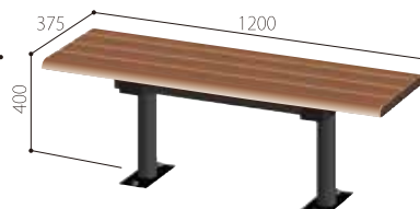
品番:DLB-90*40R-FLAT*1200-BP サイズ: W375×L1200×H400 標準価格 94,000円/基(税抜)
