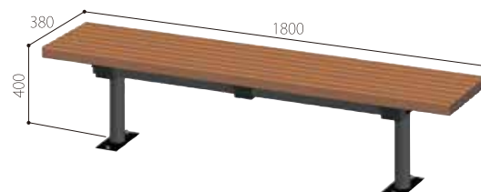
品番:DLB-50*45-FLAT-BP サイズ: W380×L1800×H400 標準価格 126,000円/基(税抜)
