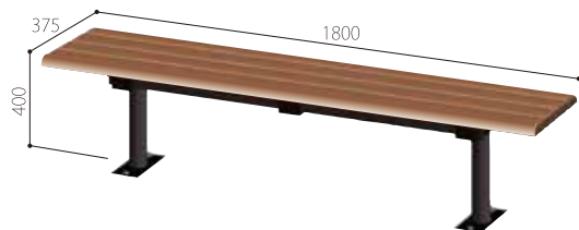
品番:DLB-90*40R-FLAT-BP サイズ: W375×L1800×H400 標準価格 108,000円/基(税抜)
