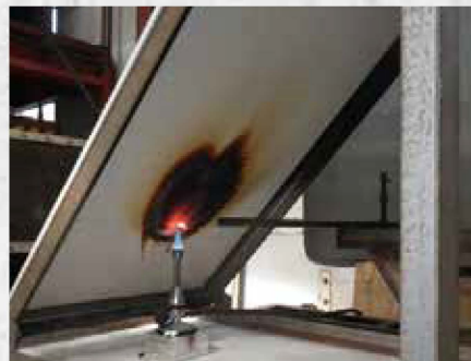
延焼性試験状況 (V1仕様)
