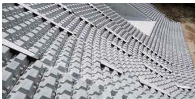
ため池護岸 ため池の護岸に用いた事例(防災タイプ)
