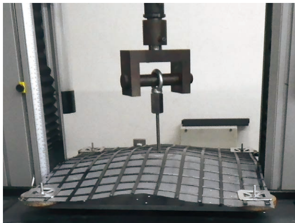
引き抜き試験状況 (HM-C11) 固定ピッチ: 500×500 mm NEXCO 小片ははく落策工の引き抜き性能規定値である0.5kN載荷時の変位が50 mm以下であることを満足しています
