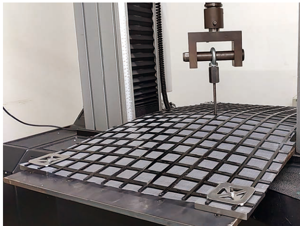
引き抜き試験状況 (HM-C22) 固定ピッチ: 900×500 mm NEXCO 小片ははく落策工の引き抜き性能規定値である0.5kN載荷時の変位が50 mm以下であることを満足しています
