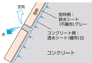
型枠側：排水シート（不織布）グレー コンクリート側：透水シート（織布）白
