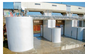
水門の施工例
