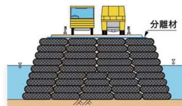
道路路体として適用する場合
