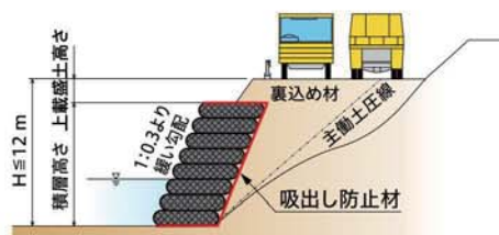
土留め構造物として適用する場合
