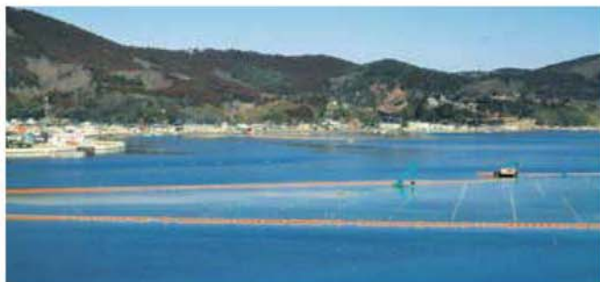
造成工事の際に汚水の流出を防いだ事例
