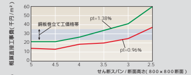
・A&P耐震補強工法の概算直接工事費と「せん断スパン/断面高さ」の関係
