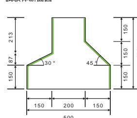
試験体断面図
