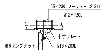
A部取付詳細図
