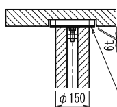
B部取付詳細図
