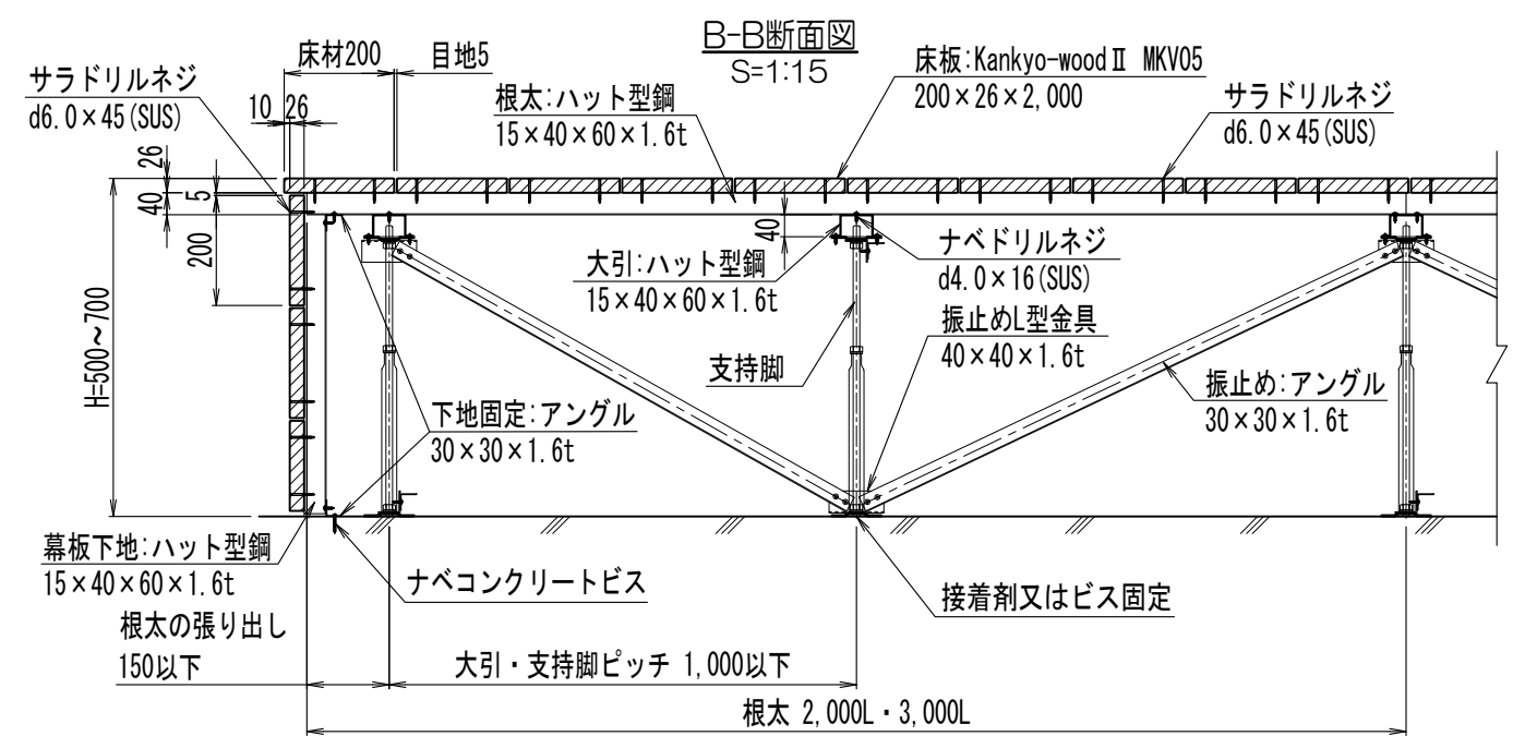
合成木材 Kankyo-wood II デッキ納まり図 MKV05 大引き・根太工法（高床仕様）
