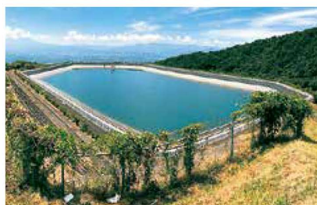
遮水工 ため池工事ににて長尺広幅シートで敷設した事例
