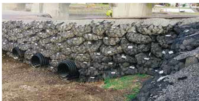
仮設工 工事用の仮設道路として用いた事例
