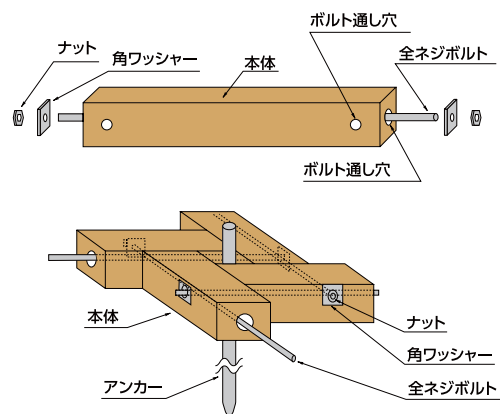
詳細図
