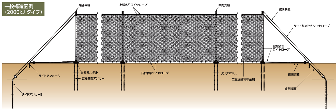
落石捕捉前
