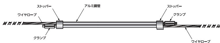
緩衝装置詳細図
