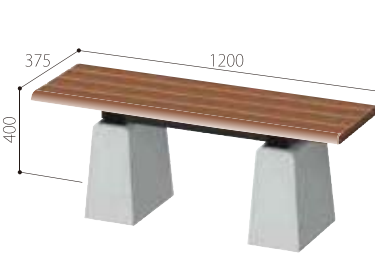
品番：DLB-90*40R-FLAT*1200-PC サイズ：W375×L1200×H400 標準価格 86,000円/基(税抜)
