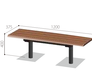
品番：DLB-90*40R-FLAT*1200 サイズ：W375×L1200×H400 標準価格 75,000円/基(税抜)
