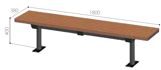
品番：DLB-50*45-FLAT-BP サイズ：W380×L1800×H400 標準価格 116,000円/基(税抜)
