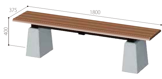
品番：DLB-90*40R-FLAT-PC サイズ：W375×L1800×H400 標準価格 97,000円/基(税抜)
