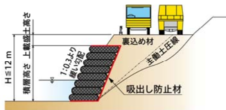
土留構造物として適用する場合
