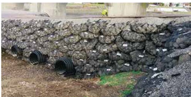
仮設工 工事用の仮設道路として用いた事例
